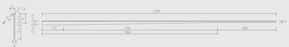
wedi Fundo Riolito neo spádový profil stěna, provedení levé
