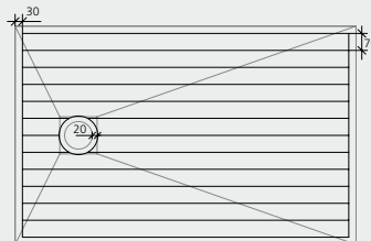
Fundo Primo 1.400 × 900 mm 2,4 × wedi 610
