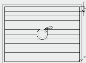
Fundo Primo 1.200 × 900 mm 2 × wedi 610
